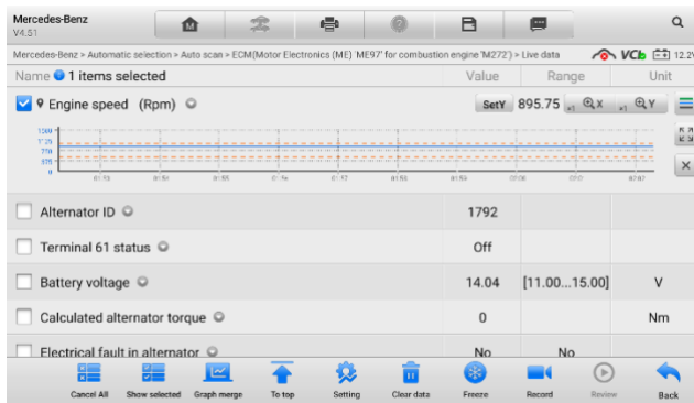
Рисунок 4-13. Пример окна для режима графика формы сигнала
