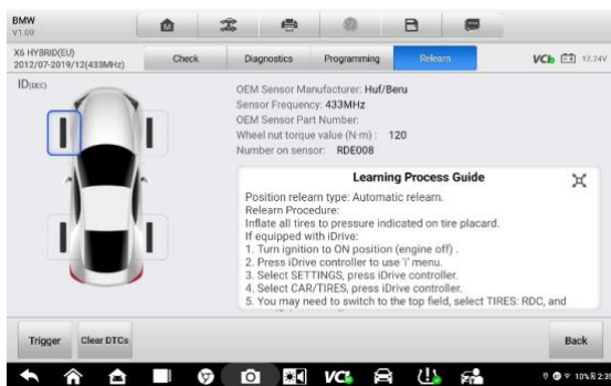
Рисунок 5-8. Пример главного окна функции повторной калибровки
