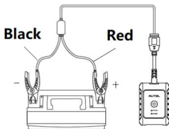
Рисунок 9-2. Подключение к автомобильному аккумулятору
